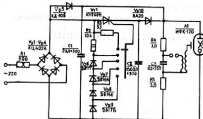
РИС. 7. СХЕМА ШИРОКОГО РЕГУЛИРОВАНИЯ ЭНЕРГИИ ВСПЫШКИ
