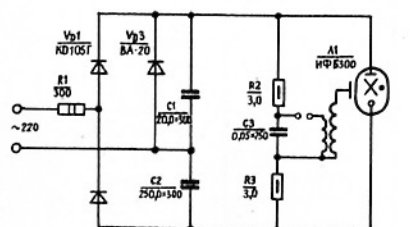
РИС. 9. СХЕМА ЗАПУСКА ЛАМПЫ ИФБ-300 ОТ СЕТИ
