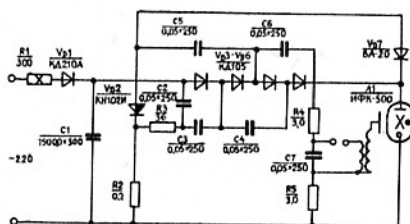
РИС. 8. СХЕМА ЗАПУСКА ВЫСОКОВОЛЬТНЫХ ЛАМП ОТ НАКОПИТЕЛЬНОЙ ЕМКОСТИ С НАПЯЖЕНИЕМ ДО 300 В
